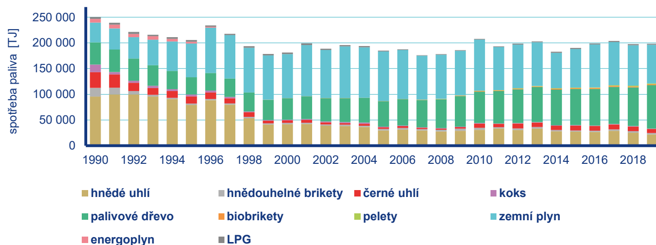
Obr. II.7 Spotřeba paliv zdrojů REZZO 3 (domácnosti), 1990–2019
