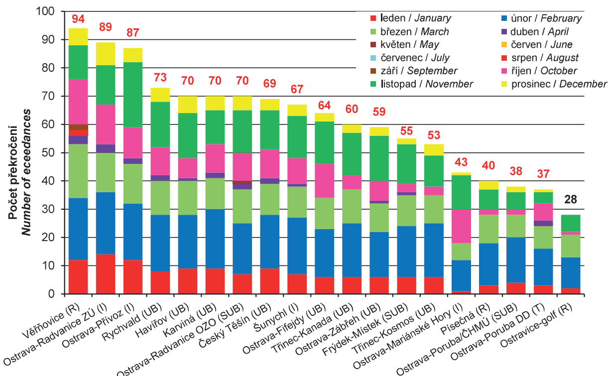
Obr. V.3.3 Počet dní s koncentracemi PM 10 > 50 µg.m -3 v jednotlivých měsících včetně celkového počtu překročení, aglomerace Ostrava/Karviná/Frydek-Místek, 2018
