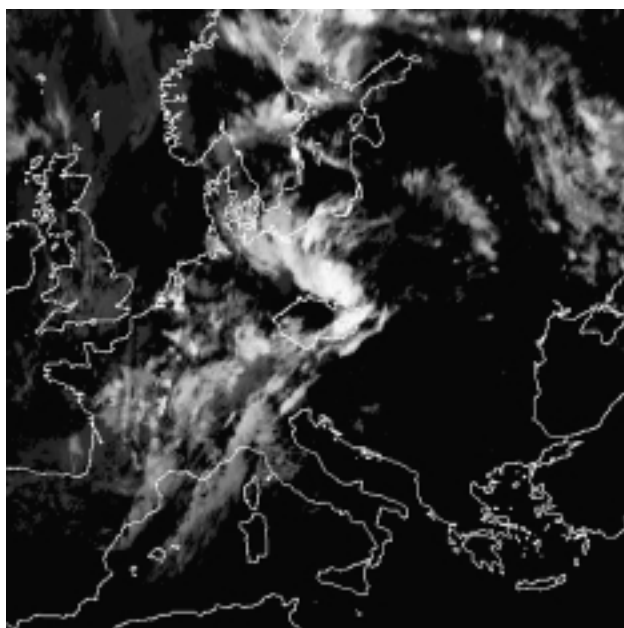
Obr. 6 Infračervený snímek družice Meteosat ze 4. 7. 1997 18 UTC.
