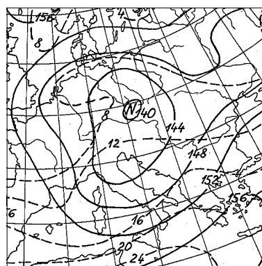
Obr. 32 Mapa hladiny 850hPa z 18. 7. 1997 12 UTC.
