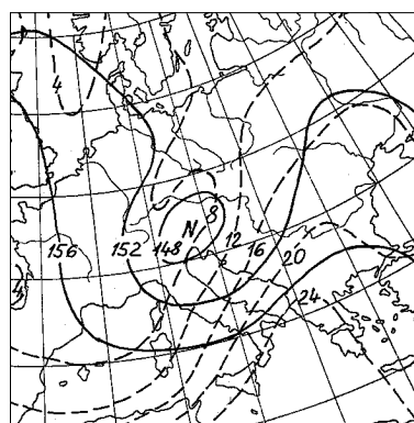
Obr. 10 Mapa hladiny 850hPa z 5. 7. 1997 12 UTC.
