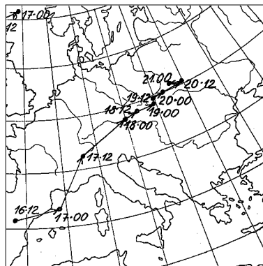
Obr. 29 Dráha středů tlakových níží na přízemních mapách od 16. 7. 1997 12UTC do 21. 7. 1997 00 UTC.
