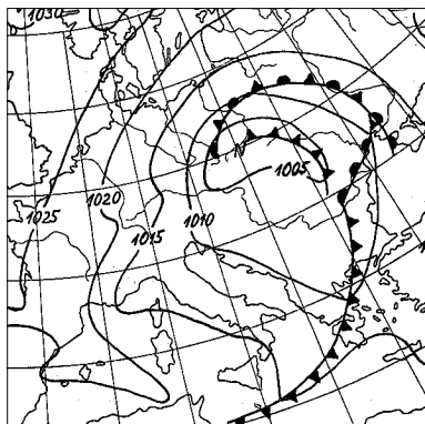
Obr. 27 Přízemní mapa z 19. 7. 1997 12 UTC.
