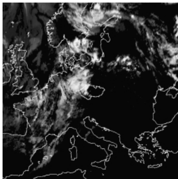
Obr. 4 Infračervený snímek družice Meteorosat ze 4. 7. 1997 12UTC.
