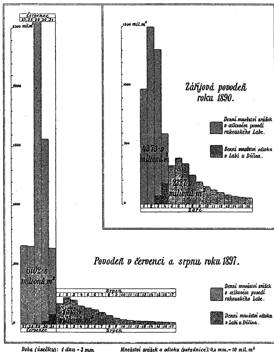
Obr. 3 Denní množství srážek [mm] a odtoku [mil. m³] v českém povodí Labe v období povodní roku 1890 a 1897 podle [22].
