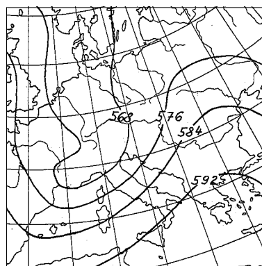
Obr. 9 Mapa hladiny 500hPa z 5. 7. 1997 12 UTC.
