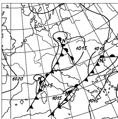
Obr. 7 Přízemní mapa ze 4. 7. 1997 18 UTC.
