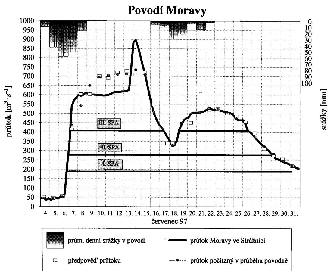
Obr. 1 Znáznornění průtoků [ \text{m}^3 \cdot \text{s}^{-1} ] a množství srážek [mm] v povodí Odry a Moravy. Fig. 1. Discharges [ \text{m}^3 \cdot \text{s}^{-1} ] and precipitation amounts [mm] in Odra and Morava basins.
