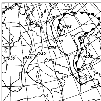
Obr. 12 Přízemní mapa z 6. 7. 1997 12 UTC. Fig. 12. Surface chart, 6 July 1997, 12 UTC.
