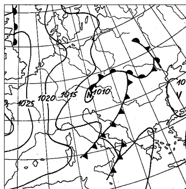
Obr. 8 Přízemní mapa z 5. 7. 1997 12 UTC.
