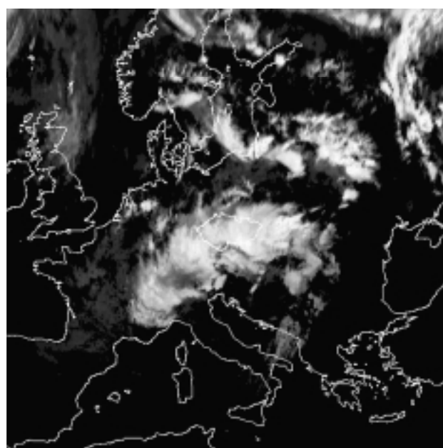
Obr. 11 Infračervený snímek družice Meteosat z 5. 7. 1997 12 UTC.
