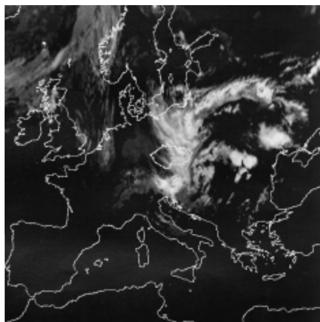
Obr. 15 Infračervený snímek družice Meteosat z 6. 7. 1997 12 UTC. Fig. 15. A Meteosat infrared picture, 6 July 1997, 12 UTC.
