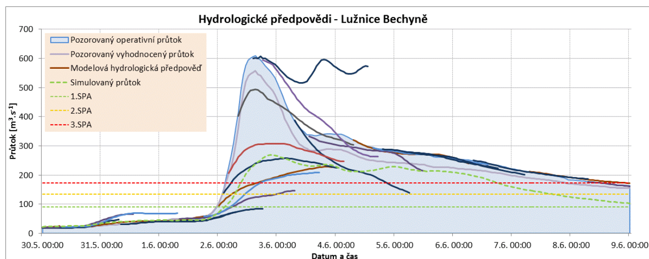
Obr. č. 13 Hydrologické předpovědi a zpětné simulace průtoku modelem podle skutečných srážek
