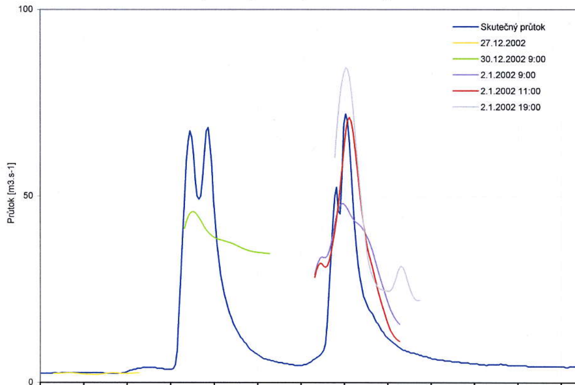
Předpovědi průtoků pro stanici Vydra - Modrava
