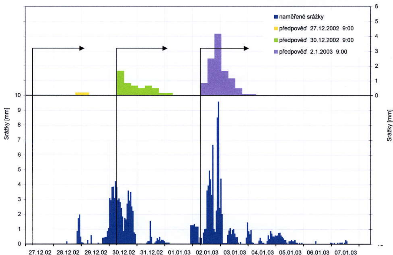
Předpovědi srážek pro povodí Vydra - Modrava a srážky vypočtené z naměřených úhrnů
