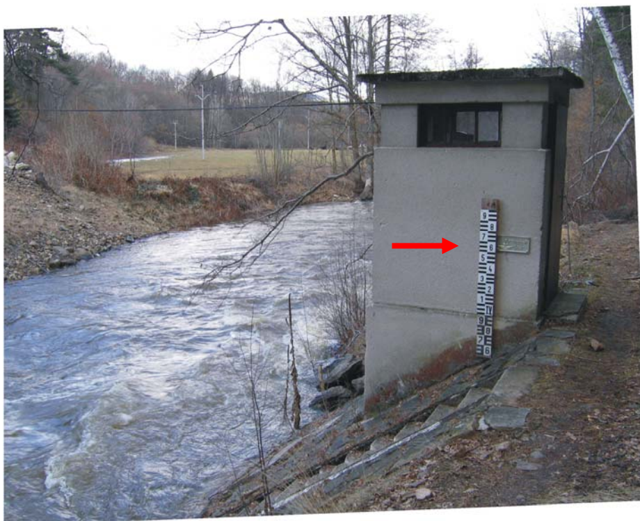
Obr. 46 Blanice, Husinec – vodočet, čtvrtek 30. března. Situace závěrové stanice Blanice, úroveň hladiny za povodně 2002 (šipka). Foto: Hovorka, P.
