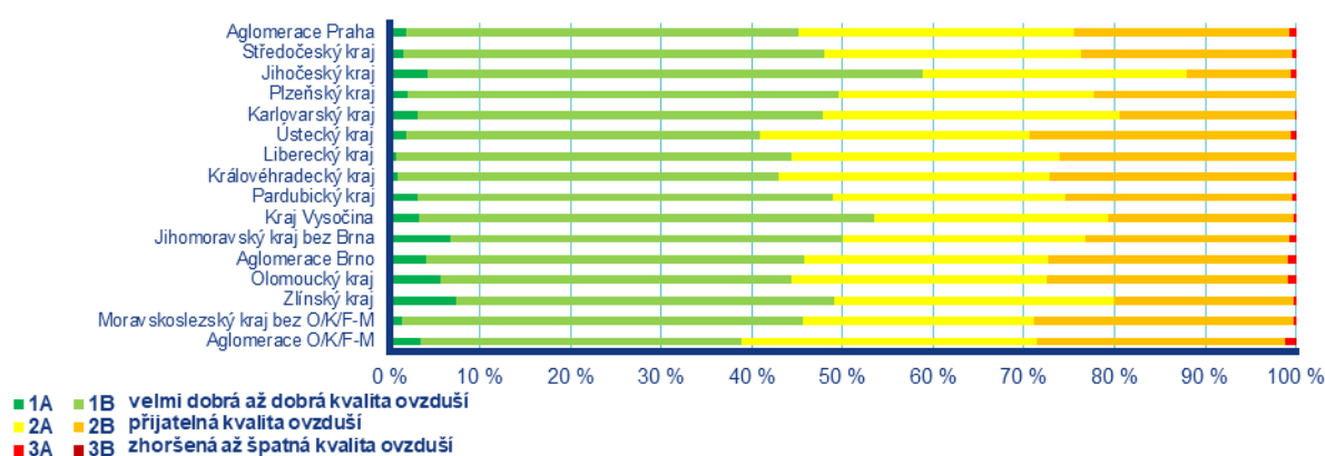
Obr. 4.6.1 Skladba indexu kvality ovzduší na městských a předměstských pozadových stanicích, září 2024
