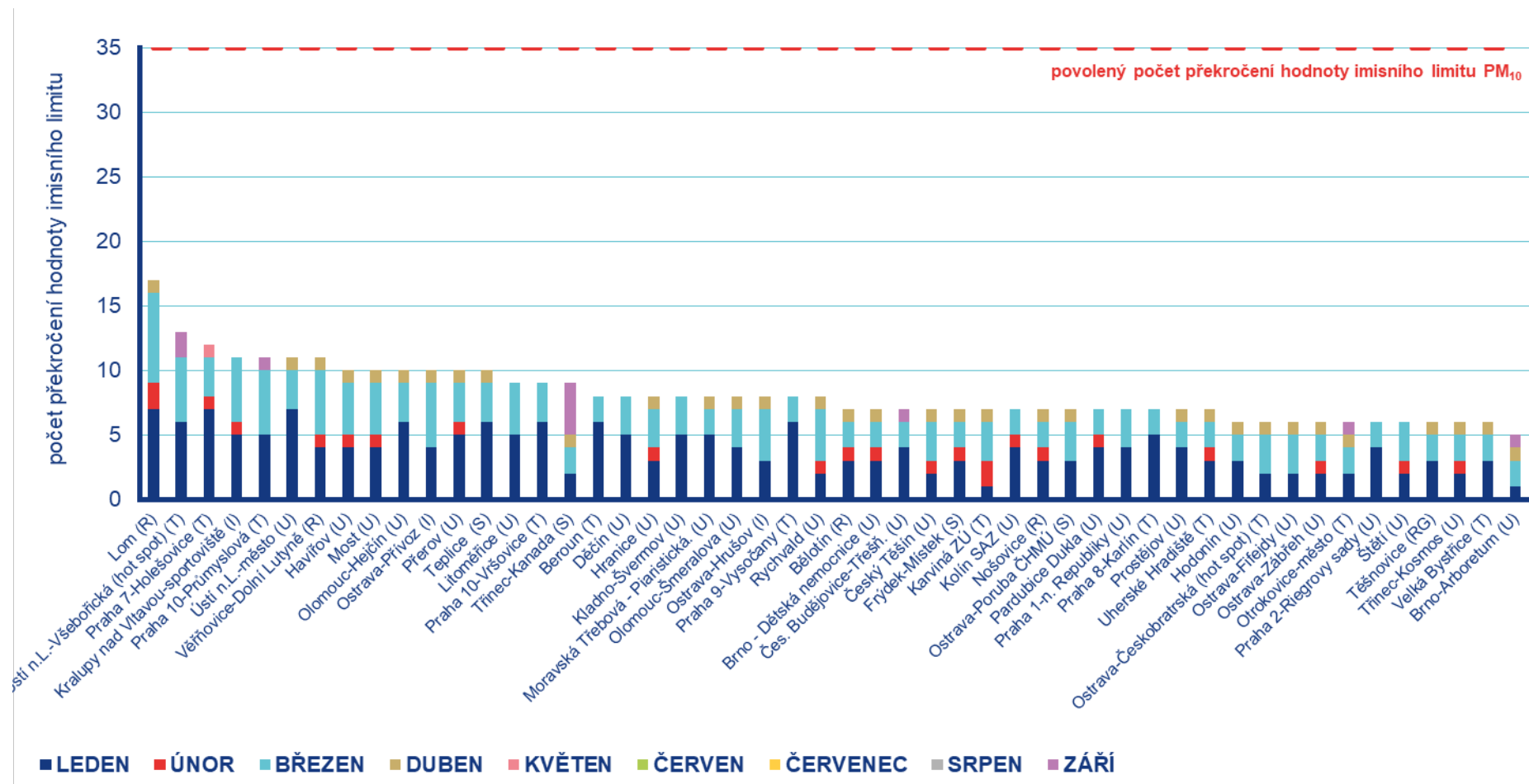
Obr. 4.2.1 Počet dnů, kdy průměrná denní koncentrace PM_{10} překročila hodnotu 24hod. imisního limitu ( 50 \mu\text{g}\cdot\text{m}^{-3} ) na stanicích AIM, 2024
