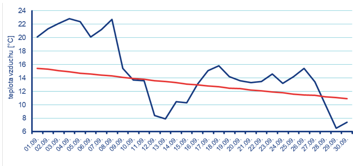
Obr. 2.1.3 Průběh průměrné denní teploty vzduchu na území ČR v září 2024 ve srovnání s normálem 1991–2020
