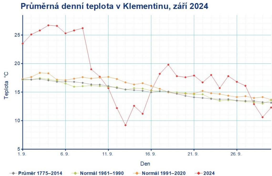
Obr. 1 Průměrná denní teplota v Praze-Klementinu v září 2024
