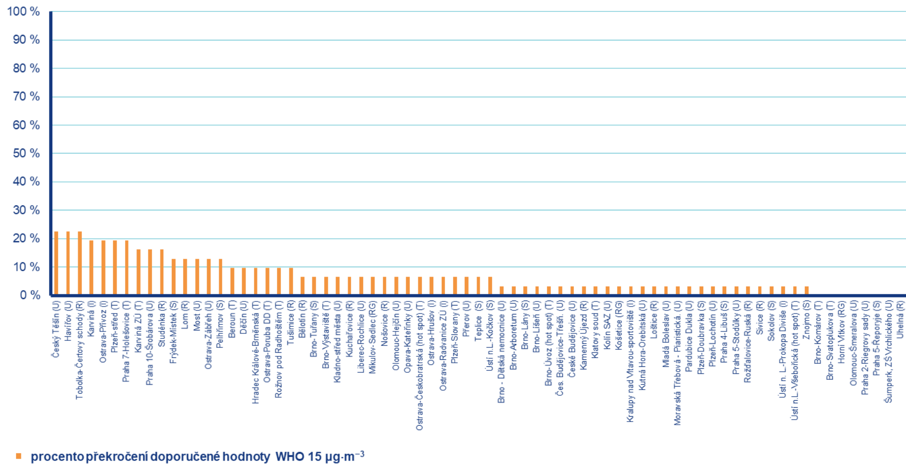
Obr. 8 Procento dní s překročením doporučené hodnoty WHO ( 15 \mu\text{g}\cdot\text{m}^{-3} ) pro průměrnou 24hodinovou koncentraci \text{PM}_{2.5} , červenec 2023
