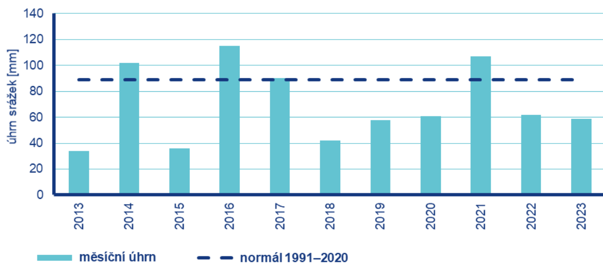
Obr. 2 Průměrný úhrn srážek v České republice, červenec 2013–2023
