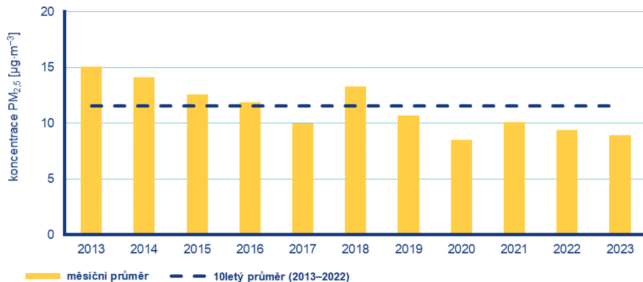
Obr. 10 Průměrné měsíční koncentrace PM_{2,5} v České republice, červenec 2013–2023
