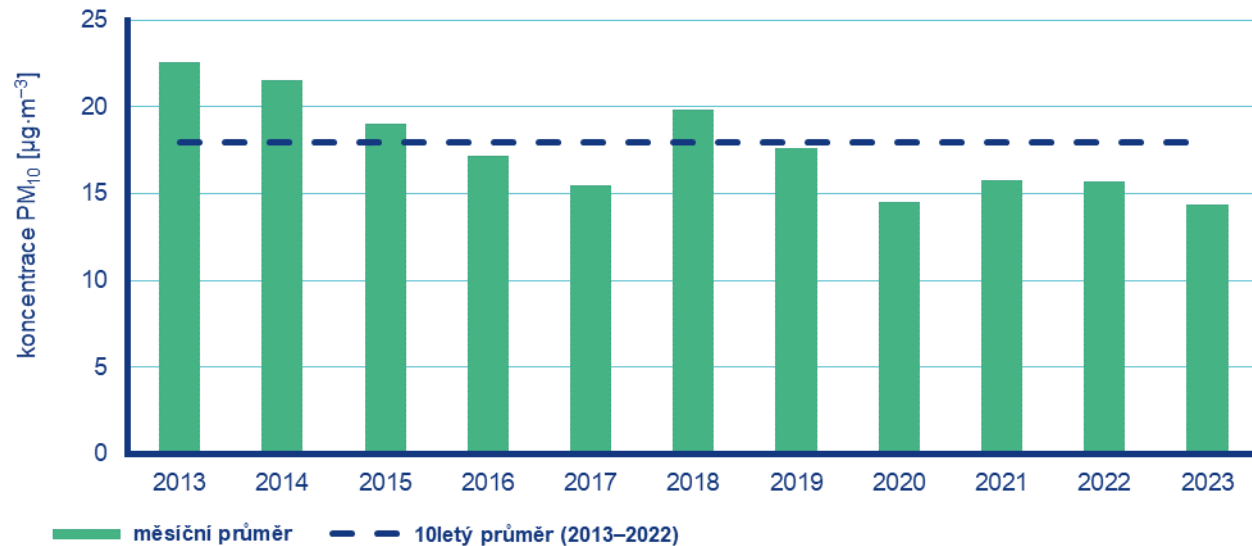
Obr. 7 Průměrné měsíční koncentrace PM_{10} v České republice, červenec 2013–2023
