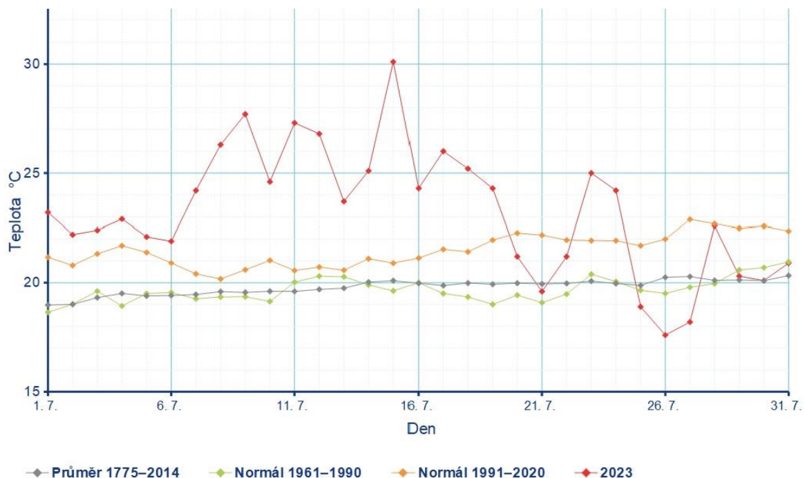
Obr. 1 Průměrná denní teplota v Praze-Klementinu v červenci 2023
