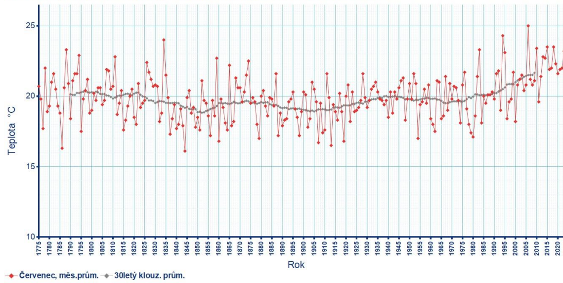
Obr. 2 Průměrná měsíční teplota v Praze-Klementinu v červenci od roku 1775 do roku 2023
