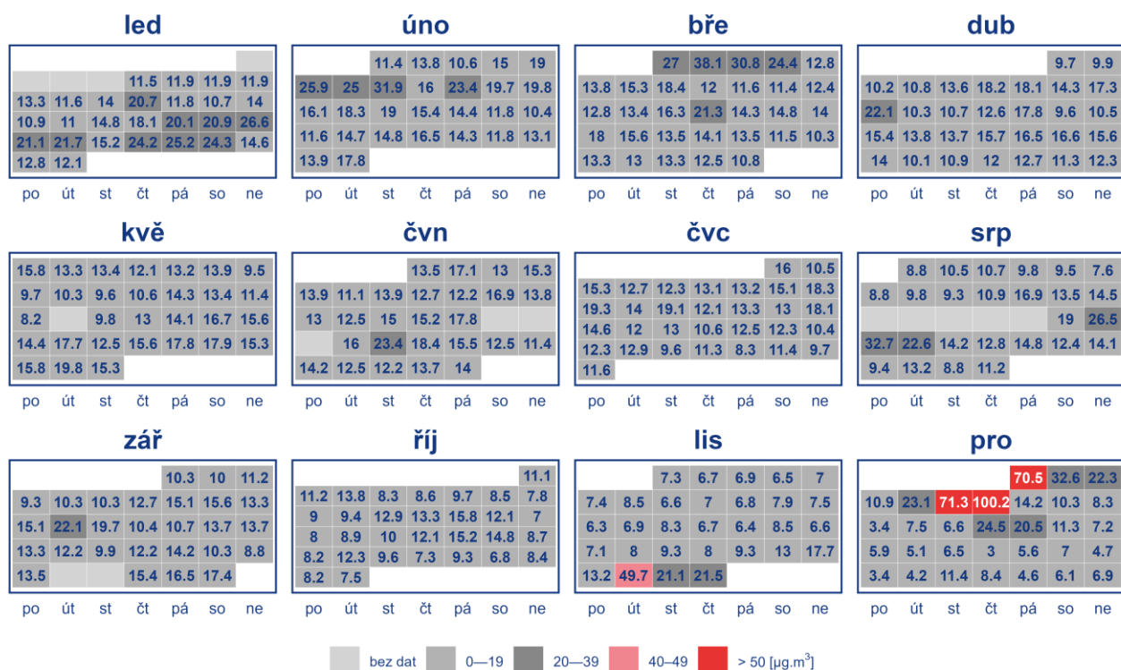
Obr. 7 Průměrné denní koncentrace PM 10 na stanici Morávka, 2023
