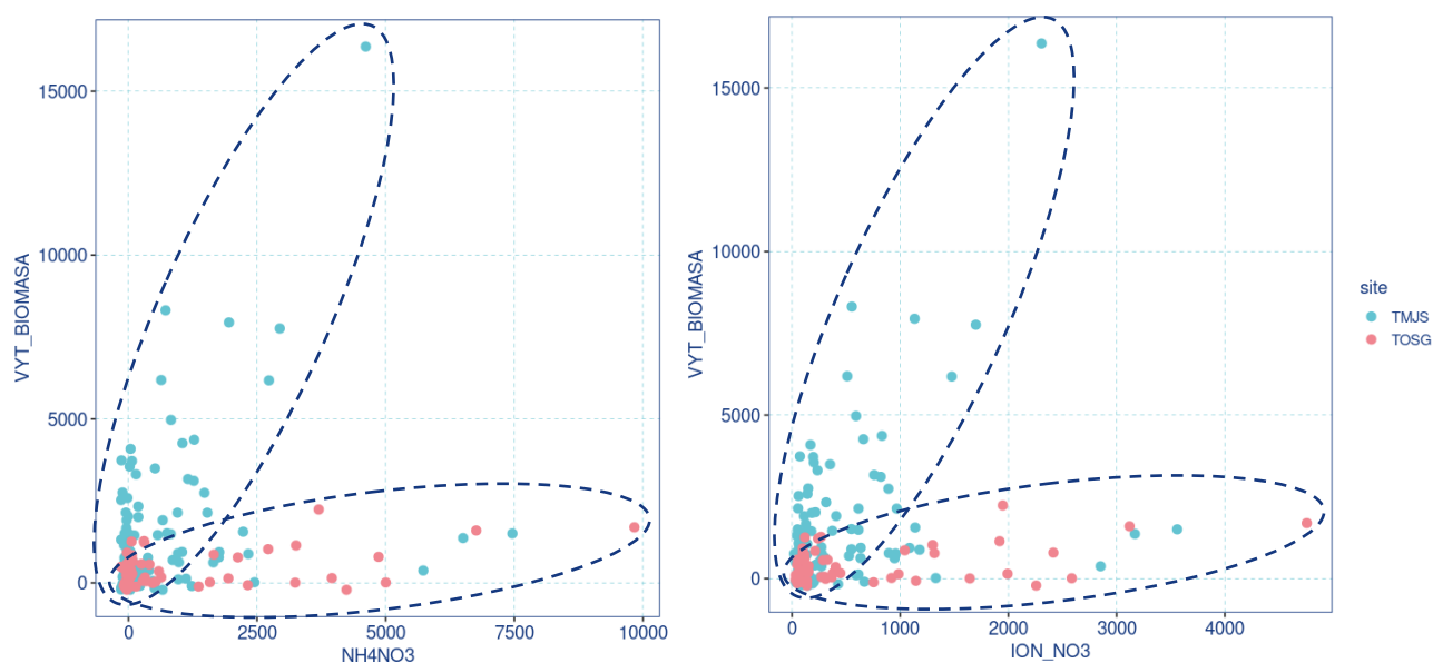
Obr. 22 Souvislost mezi vytápěním biomasou a dusičnany [ \text{ng.m}^{-3} ]; vlevo vztah mezi modelovaným příspěvkem vytápění biomasou a modelovaným příspěvkem dusičnanu amonného, vpravo vztah mezi modelovaným příspěvkem vytápění biomasou a skutečně naměřenou koncentrací dusičnanů.
