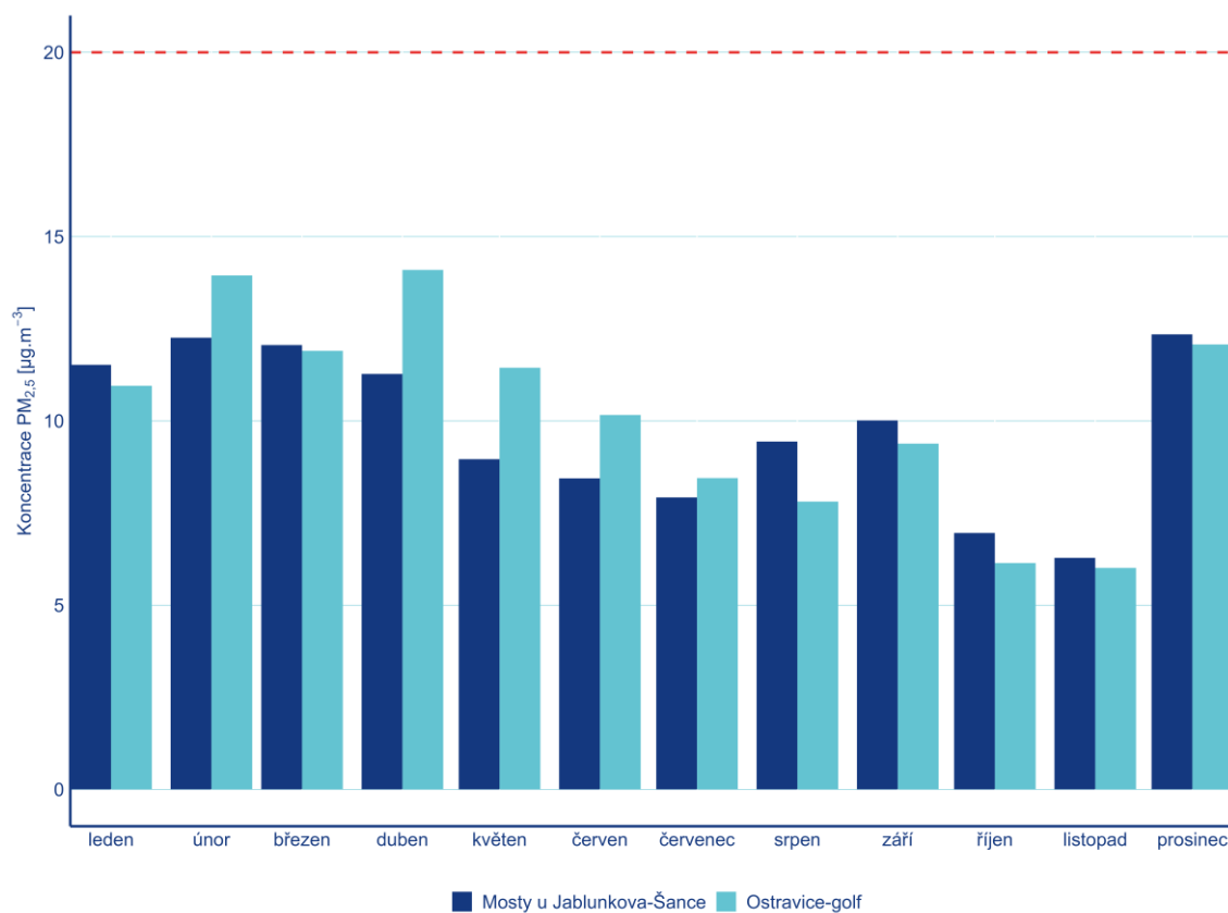
Obr. 5 Roční chod průměrných měsíčních koncentrací PM_{2.5} , 2023
