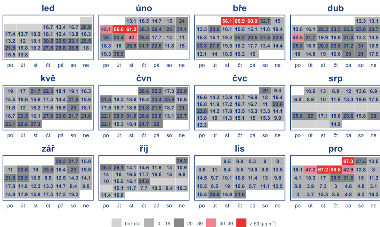
Obr. 6 Průměrné denní koncentrace PM 10 na stanici Metylovice, 2023
