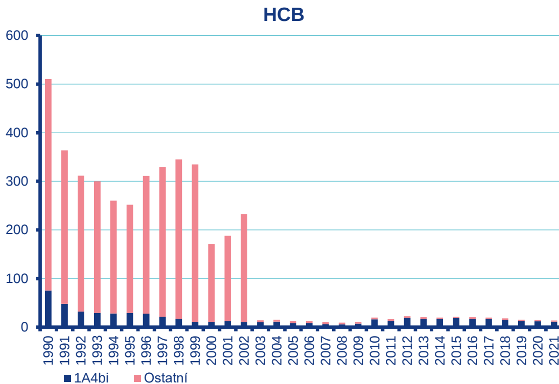
Obr. C7 – Vývoj emisí HCB sektoru 1A4bi a celkových emisí HCB, 1990–2021
