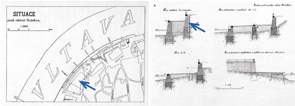
Obr. 6 Projekt nově budovaného nábřeží v r. 1900 s vyznačením limnigrafu pod Rudolfinem a řezy s vyznačením jeho šachty (Erben, Srb 1904).
