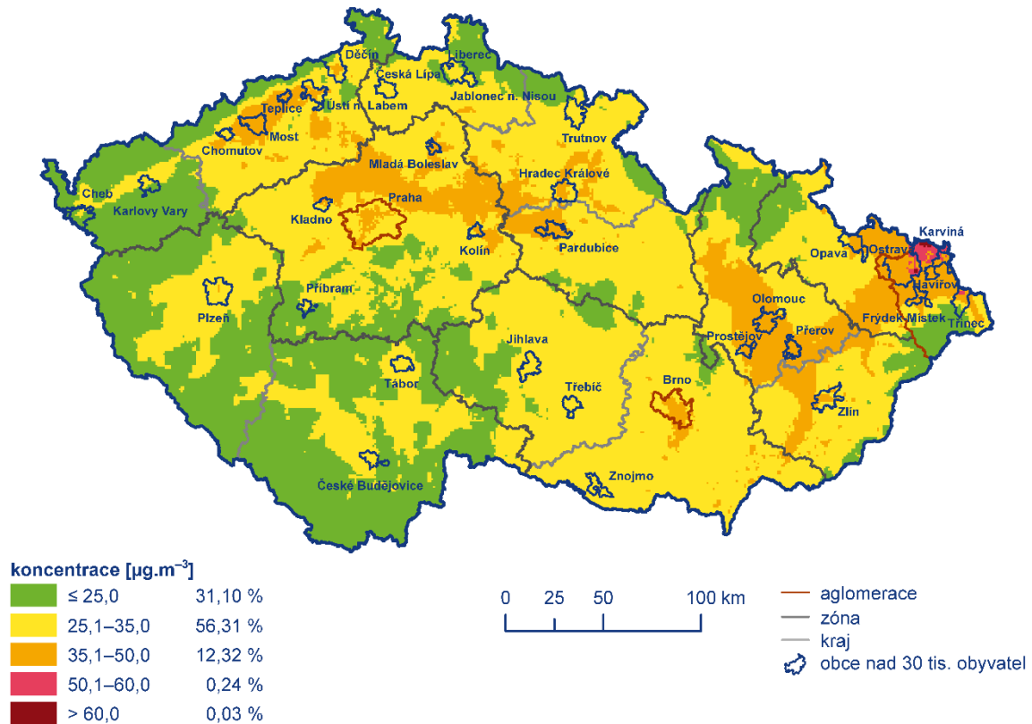
Obr. 5 Pole 36. nejvyšší 24hod. koncentrace PM_{10} , 2019
