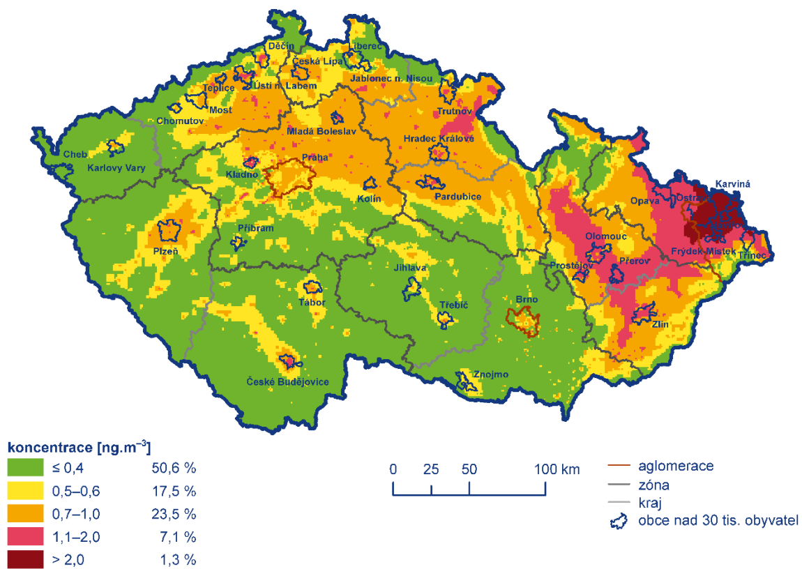
Obr. 6b Pole roční průměrné koncentrace benzo[a]pyrenu, 2019
