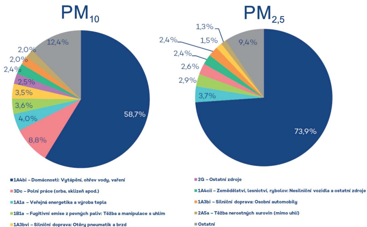
Obr. 9 Podíl sektorů NFR na celkových emisích PM 10 a PM 2,5 , 2018
