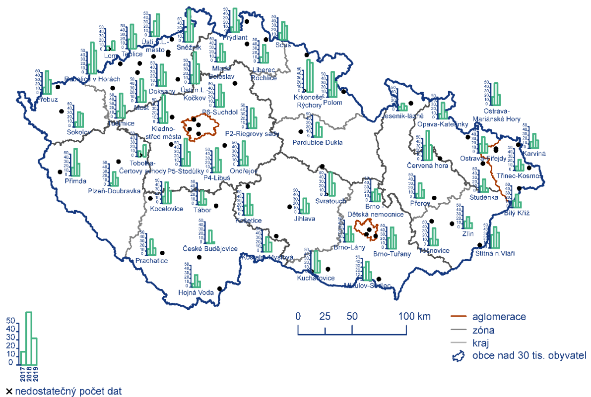
Obr. 7a Počet překročení 8hod. imisního limitu přízemního ozonu za rok na vybraných stanicích, 2017–2019
