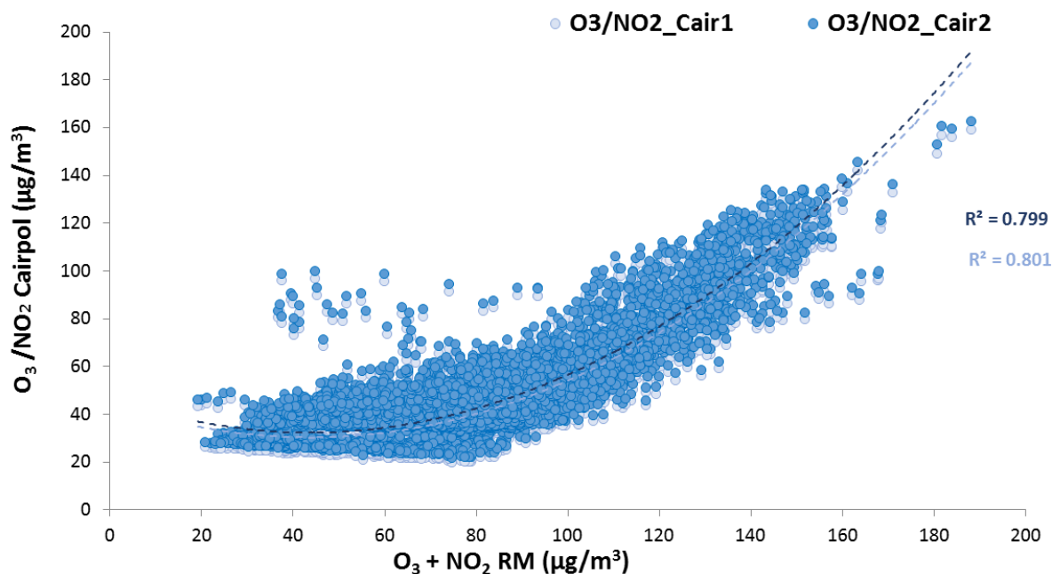
Obr. č. 4. Porovnání hodinových koncentrací O 3 a NO 2 naměřených kombinovanými Cairpol senzory (osa y; O 3 /NO 2 _Cair1 a O 3 /NO 2 _Cair2) a RM (osa x). R 2 = koeficient determinace vycházející z nelineární rovnice vztahu mezi hodnotami naměřenými senzory a RM.
