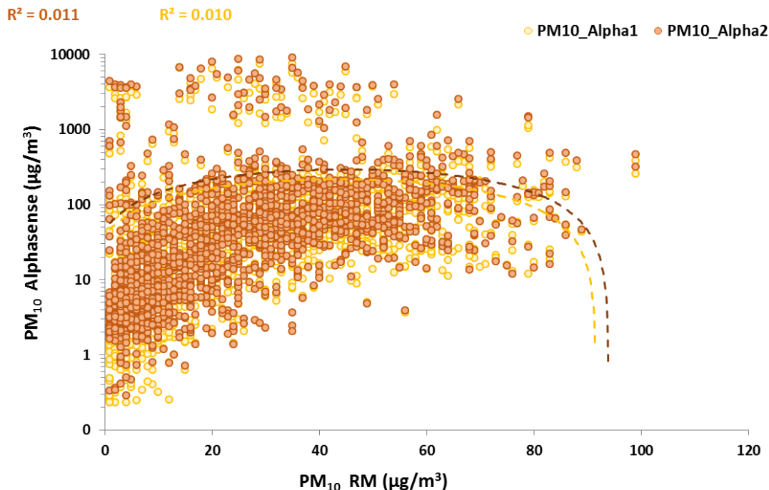
Obr. č. 23. Porovnání hodinových koncentrací částic PM_{10} naměřených Alphasense senzory (osa y; PM_{10\_Alpha1} a PM_{10\_Alpha2} ) a RM (osa x). R^2 = koeficient determinace vycházející z nelineární rovnice vztahu mezi hodnotami naměřenými senzory a RM. Osa y je zobrazena v logaritmické škále.
