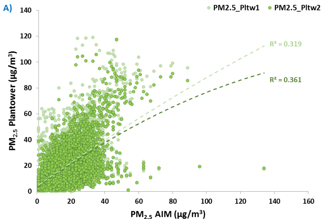
Obr. č. 10. Porovnání hodinových koncentrací částic PM_{2.5} naměřených Plantower senzory (osa y; PM_{2.5\_Pltw1} a PM_{2.5\_Pltw2} ) a RM (osa x). R^2 = koeficient determinace vycházející z nelineární rovnice vztahu mezi hodnotami naměřenými senzory a RM.
