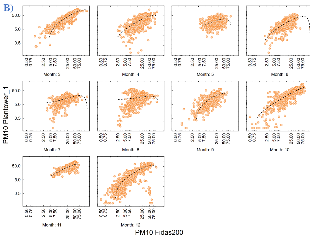
Obr. č. 19. Porovnání hodinových koncentrací PM 10 naměřených Plantower_1 senzorem (osa y) a A) RM (osa x), B) nereferenčním Fidas200 analyzátořem (osa x) v jednotlivých měsících měřicího období. Koncentrace jsou udány v \mu\text{g}/\text{m}^3 . Osy x a y jsou zobrazeny v logaritmické škále.
