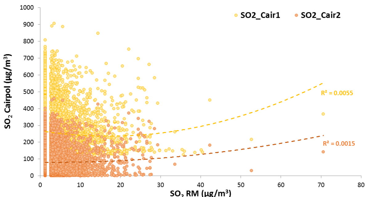
Obr. č. 3. Porovnání hodinových koncentrací SO 2 naměřených Cairpol senzory (osa y; žlutě SO 2 _Cair1 a oranžově SO 2 _Cair2) a referenčním monitorem AIM stanice (osa x). R 2 = koeficient determinace vycházející z nelineární rovnice vztahu mezi hodnotami naměřenými senzory a RM.
