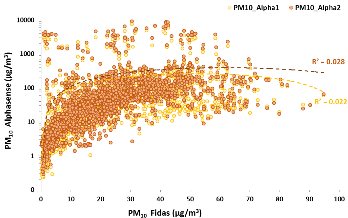
Obr. č. 26. Porovnání hodinových koncentrací částic PM_{10} naměřených Alphasense senzory (osa y; PM_{10\_Alpha1} a PM_{10\_Alpha2} ) a nereferenčním analyzátořem Fidas200 (osa x). R^2 = koeficient determinace vycházející z nelineární rovnice vztahu mezi hodnotami naměřenými senzory a Fidas analyzátořem. Osa y je zobrazena v logaritmické škále.
