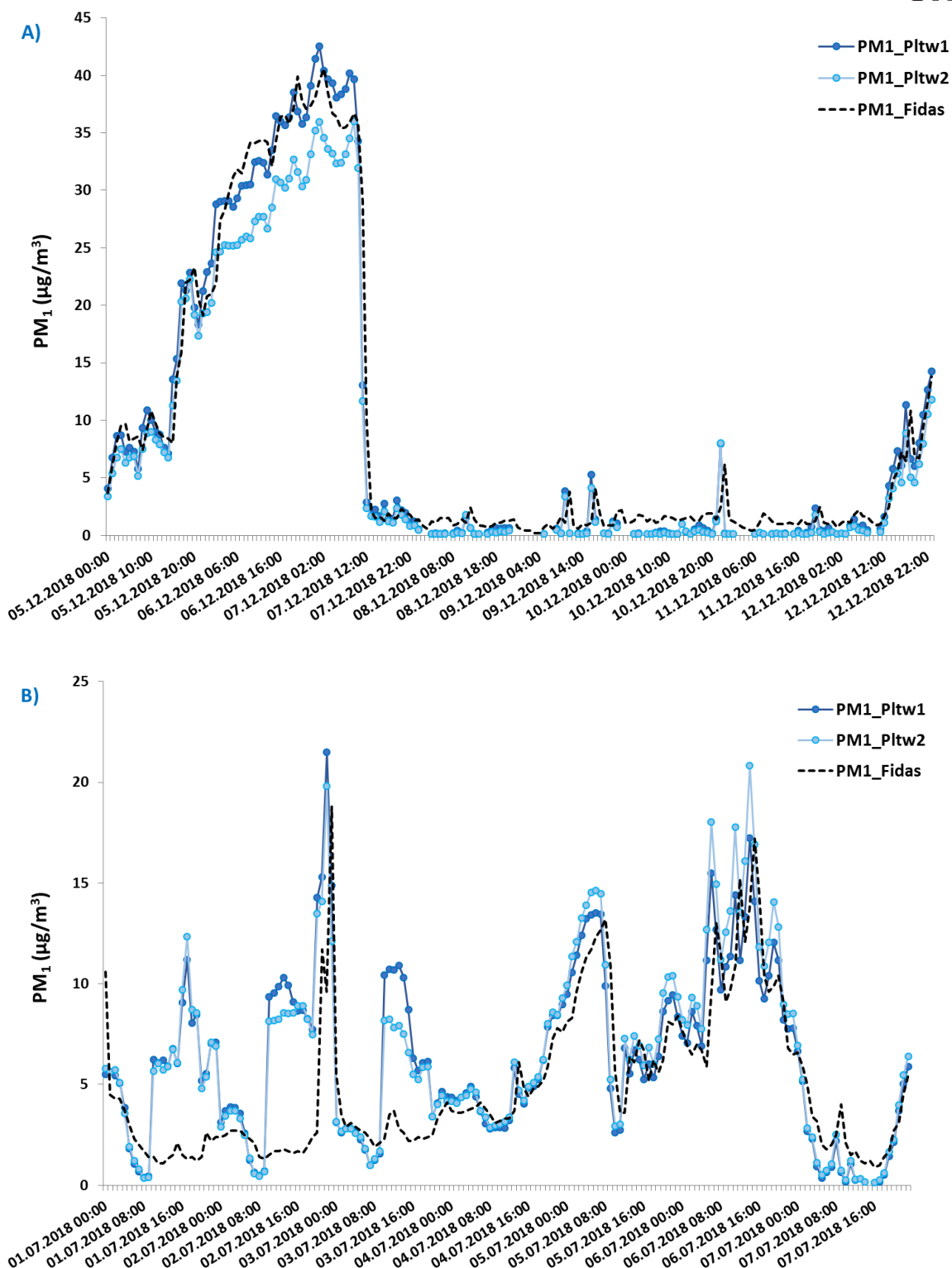
Obr. č. 15. Průběh hodinových koncentrací částic PM 1 naměřených Plantower senzory (Pltw1, Pltw2; plné čáry) a nereferenčním analyzátořem Fidas200 (přerušovaná čára) A) v zimním období od 5.12. do 12.12. 2018, B) v letním období od 1.7. do 7.7. 2018.
