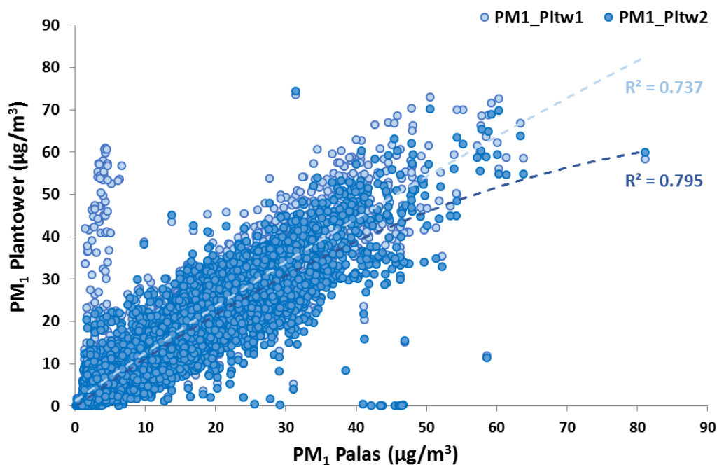
Obr. č. 12. Porovnání hodinových koncentrací částic PM_1 naměřených Plantower senzory (osa y; PM_1\_Pltw1, PM_1\_Pltw2 ) a analyzátořem Palas Fidas200 (osa x). R^2 = koeficient determinace vycházející z nelineární rovnice vztahu mezi hodnotami naměřenými senzory a analyzátořem Fidas200.
