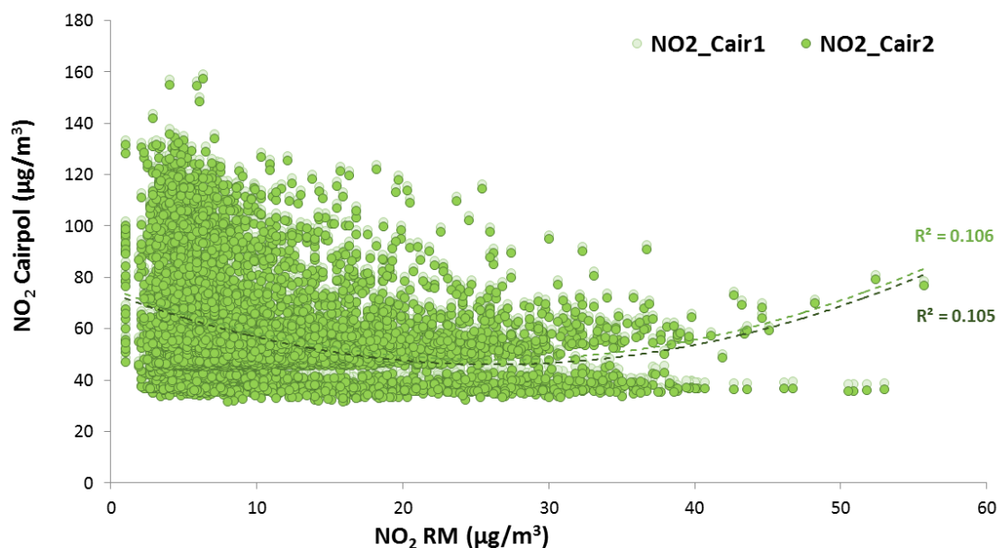
Obr. č. 5. Porovnání hodinových koncentrací NO 2 naměřených samostatnými Cairpol senzory (osa y; NO 2 _Cair1, NO 2 _Cair2) a RM (osa x). R 2 = koeficient determinace vycházející z nelineární rovnice vztahu mezi hodnotami naměřenými senzory a RM.
