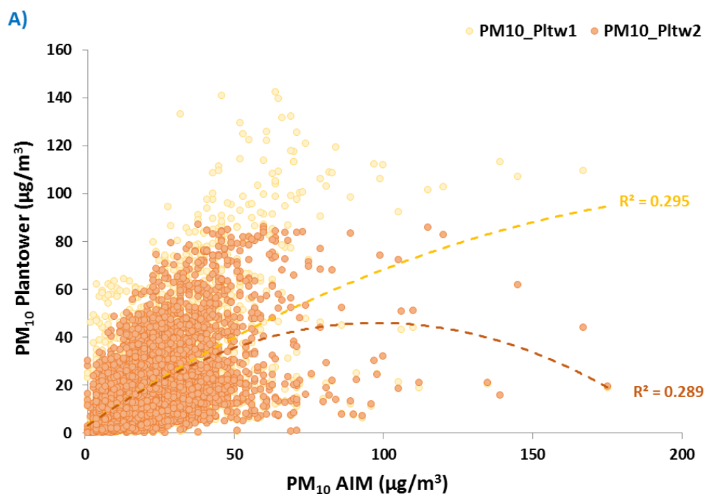
Obr. č. 11. Porovnání hodinových koncentrací částic PM_{10} naměřených Plantower senzory (osa y; PM_{10\_Pltw1} a PM_{10\_Pltw2} ) a RM (osa x). R^2 = koeficient determinace vycházející z nelineární rovnice vztahu mezi hodnotami naměřenými senzory a RM.
