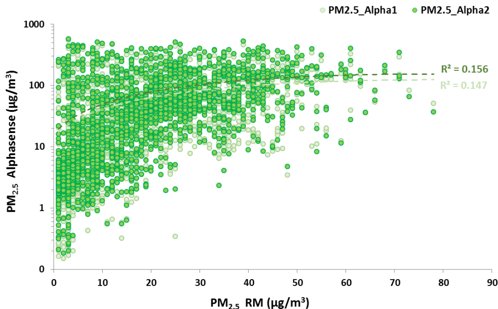
Obr. č. 22. Porovnání hodinových koncentrací částic PM_{2.5} naměřených Alphasense senzory (osa y; PM_{2.5\_Alpha1} a PM_{2.5\_Alpha2} ) a RM (osa x). R^2 = koeficient determinace vycházející z nelineární rovnice vztahu mezi hodnotami naměřenými senzory a RM. Osa y je zobrazena v logaritmické škále.
