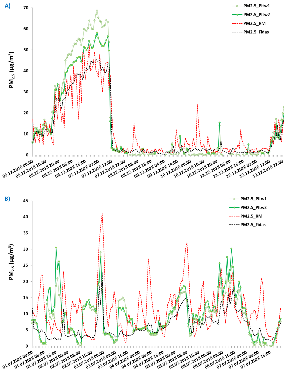
Obř. ř. 16. Průběh hodinových koncentrací částic PM 2.5 naměřených Plantower senzory (Pltw1, Pltw2; plné čáry), RM a nereferenčním analyzátořem Fidas200 (přerušované čáry) A) v zimním období od 5.12. do 12.12.2018, B) v letním období od 1.7. do 7.7. 2018.
