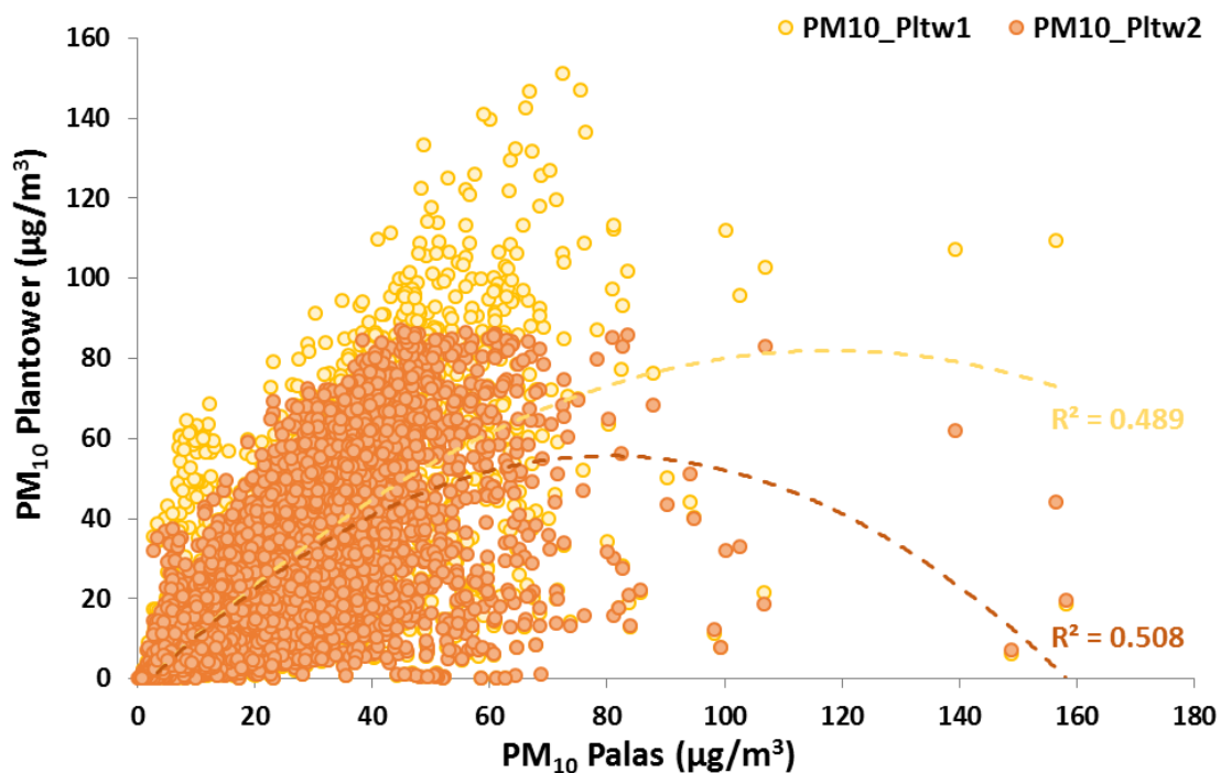
Obr. č. 14. Porovnání hodinových koncentrací částic PM 10 naměřených Plantower senzory (osa y; PM 10 _Pltw1, PM 10 _Pltw2) a analyzátořem Palas Fidas200 (osa x). R 2 = koeficient determinace vycházející z nelineární rovnice vztahu mezi hodnotami naměřenými senzory a analyzátořem Fidas200.
