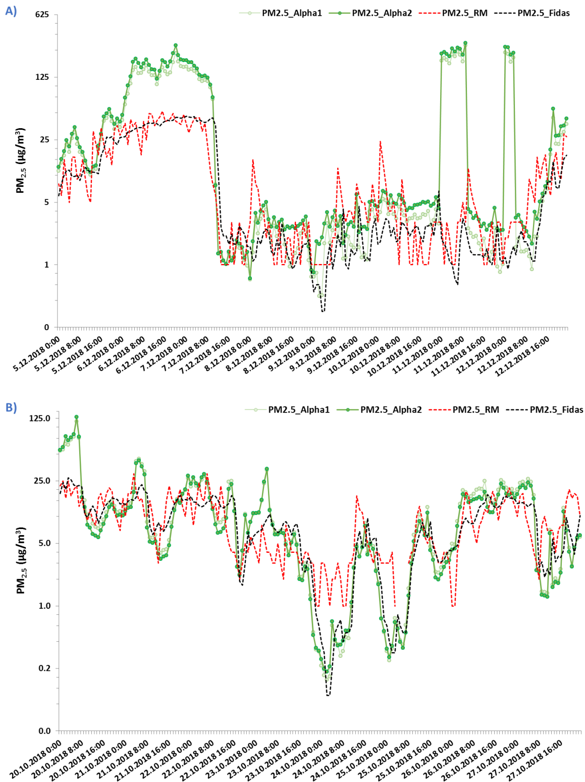
Obr. č. 28. Průběh hodinových koncentrací částic PM_{2.5} naměřených Alphasense senzory (Alpha1, Alpha2; osa y; plné čáry), RM a nereferečním analyzátořem Fidas200 (osa y; přerušované čáry) A) v zimním období od 5.12. do 12.12. 2018, B) v podzimním období od 20.10. do 27.10. 2018. Osy y jsou zobrazeny v logaritmické škále.
