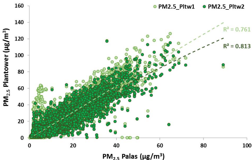
Obr. č. 13. Porovnání hodinových koncentrací částic PM_{2.5} naměřených Plantower senzory (osa y; PM_{2.5\_Pltw1}, PM_{2.5\_Pltw2} ) a analyzátořem Palas Fidas200 (osa x). R^2 = koeficient
