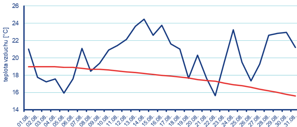
Obr. 2.1.3 Průběh průměrné denní teploty na území ČR v srpnu 2024 ve srovnání s normálem 1991–2020
