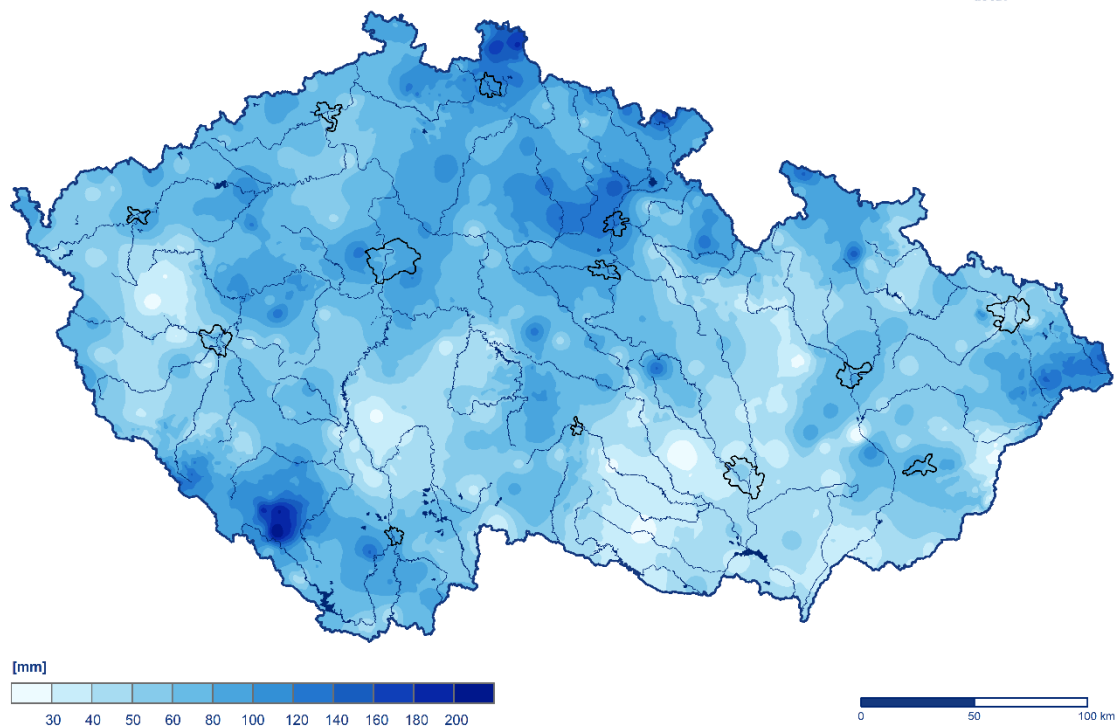
Obr. 2.2.1 Měsíční úhrn srážek na území ČR v srpnu 2024
