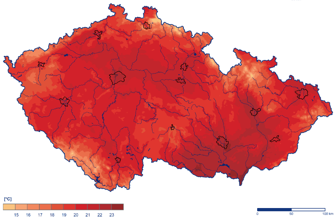
Obr. 2.1.1 Průměrná měsíční teplota vzduchu na území ČR v srpnu 2024
