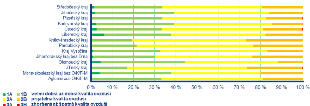
Obr. 4.6.2 Skladba indexu kvality ovzduší na venkovských pozad'ových stanicích, srpen 2024
