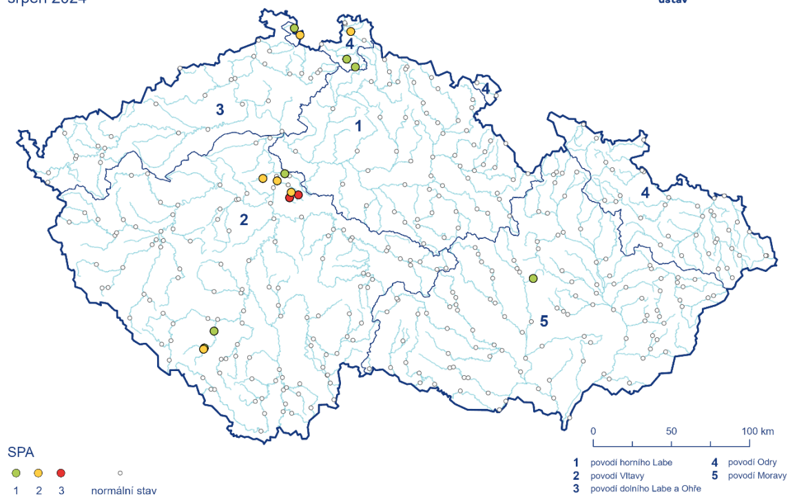
Obr. 3.1.4 Dosažené stupně povodňové aktivity, srpen 2024
