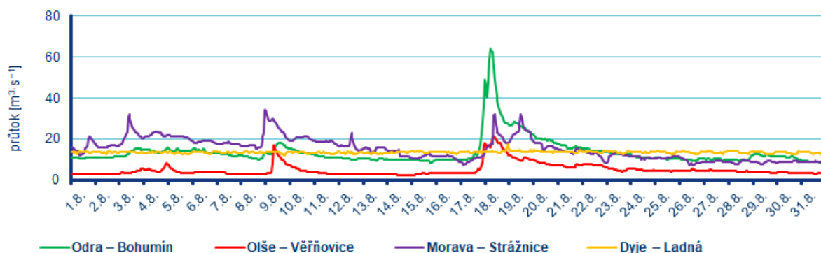
Obr. 3.1.2 Průběh průtoků v závěrových profilech Odry, Olše, Moravy a Dyje, srpen 2024
