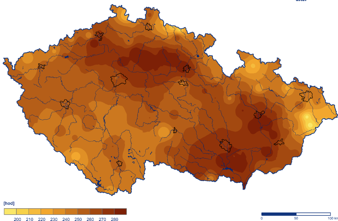
Obr. 2.3.1 Měsíční úhm doby trvání slunečního svitu na území ČR v srpnu 2024
