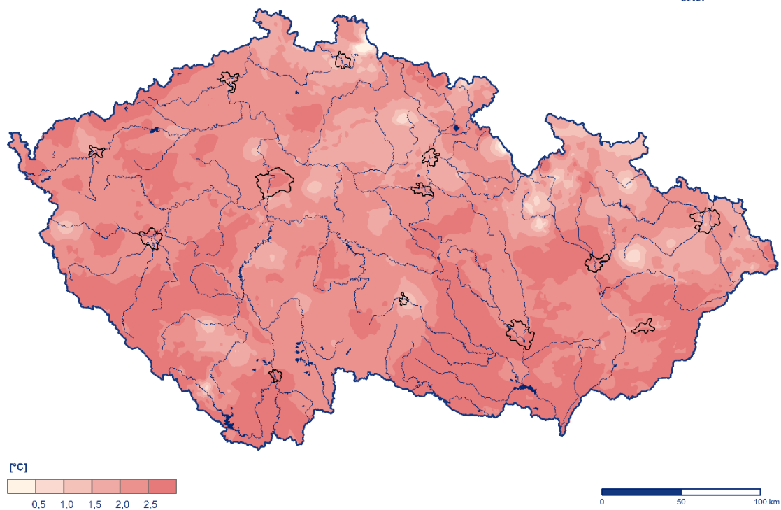
Obr. 2.1.2 Odchylka průměrné měsíční teploty vzduchu od normálu 1991–2020 na území ČR v srpnu 2024
